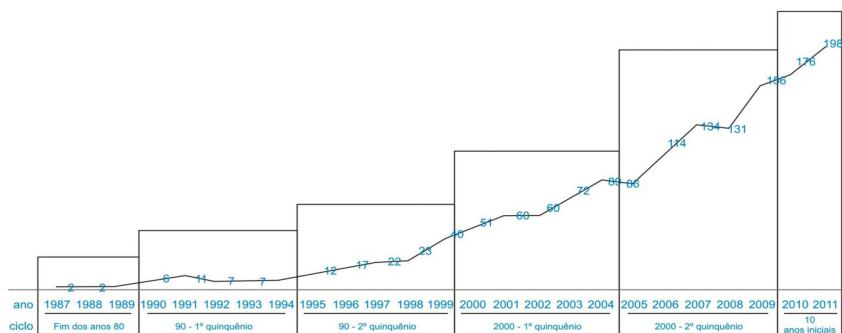
Gráfico1 - Distribuição da produção stricto sensu sobre pessoa com deficiência por ano
