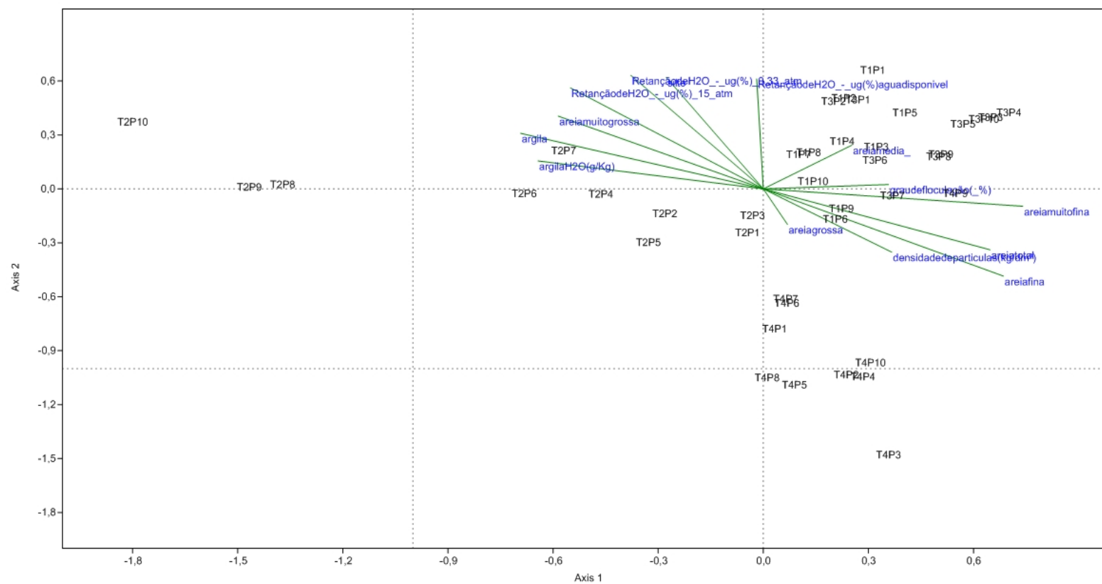
Figura 2. Gráfico de análise canônica para química do solo com relação à distribuição das parcelas.
