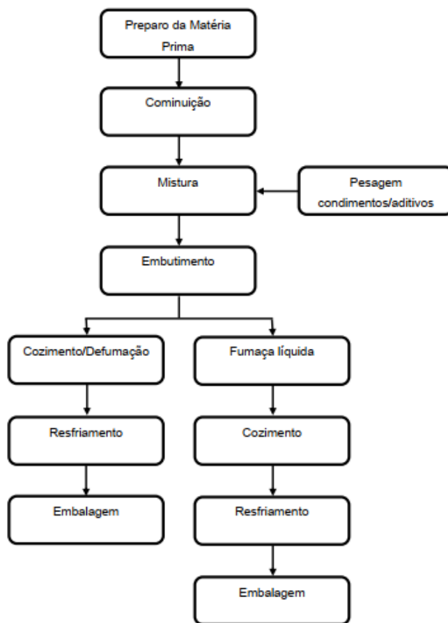
Figura 9 - Fluxograma do processo de defumação de linguiça
