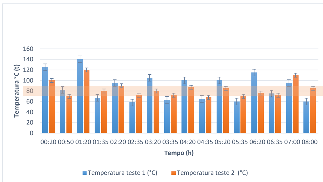
Figura 21 - Gráfico de variações de temperatura no teste 1 e no teste 2
