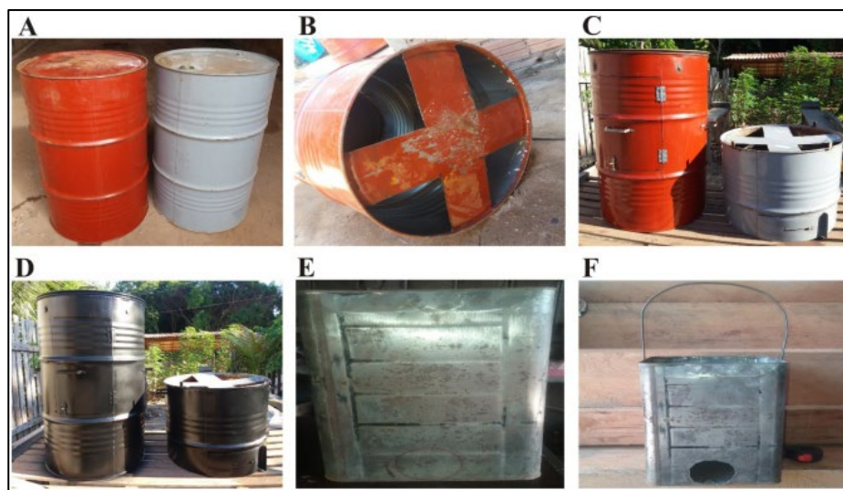
Figura 12 - Processo de construção do defumador caseiro
