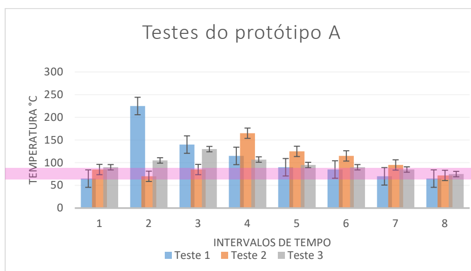
Figura 20 - Gráfico do perfil comparativo de temperaturas obtidos nos testes com o Protótipo A
