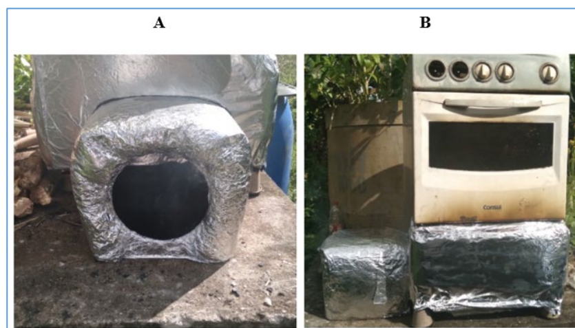
Figura 18 - Protótipo B montado para o teste 2
