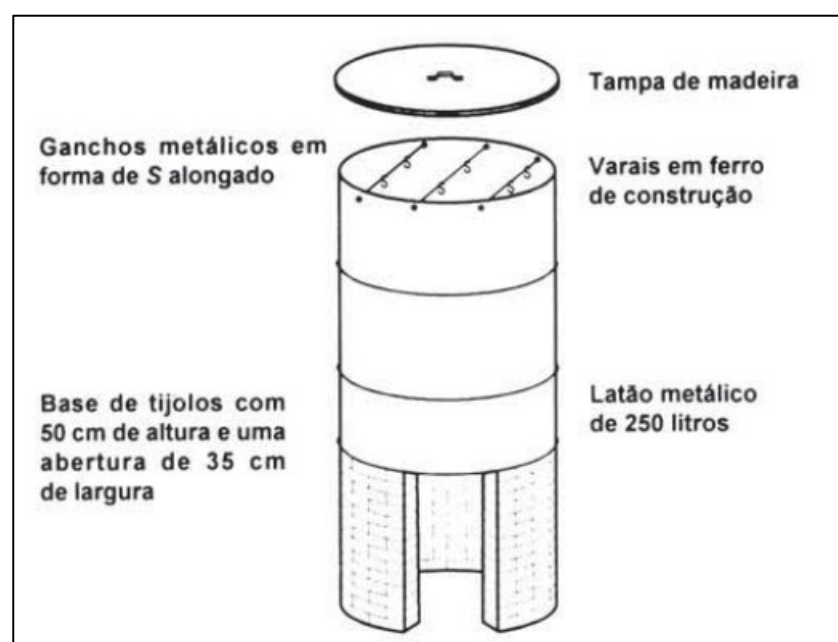
Figura 2 - Processo de defumação a quente
