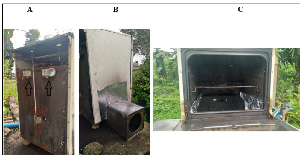
Figura 17 - Protótipo B montado para o teste 1
