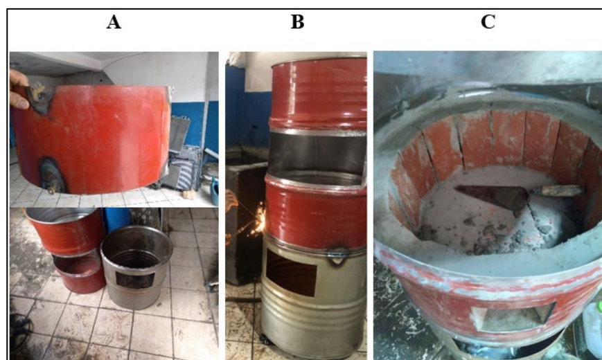
Figura 13 - Etapas de fabricação do defumador: (A) tambores utilizados; (B) detalhe do processo de soldagem do defumador; (C) detalhes do revestimento refratário
