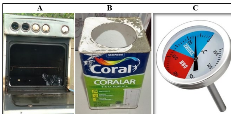
Figura 16 - Materiais para fabricação do protótipo B: (A) fogão doméstico inutilizado; (B) lata usada de tinta; (C) termômetro analógico de defumador
