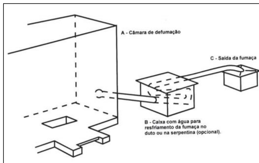
Figura 1 - Processo de defumação a frio
