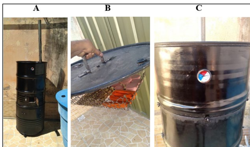
Figura 15 - Etapas de fabricação do defumador: (A) Protótipo A finalizado com a instalação da chaminé; (B) cesto para acomodação das carnes (C) termômetro
