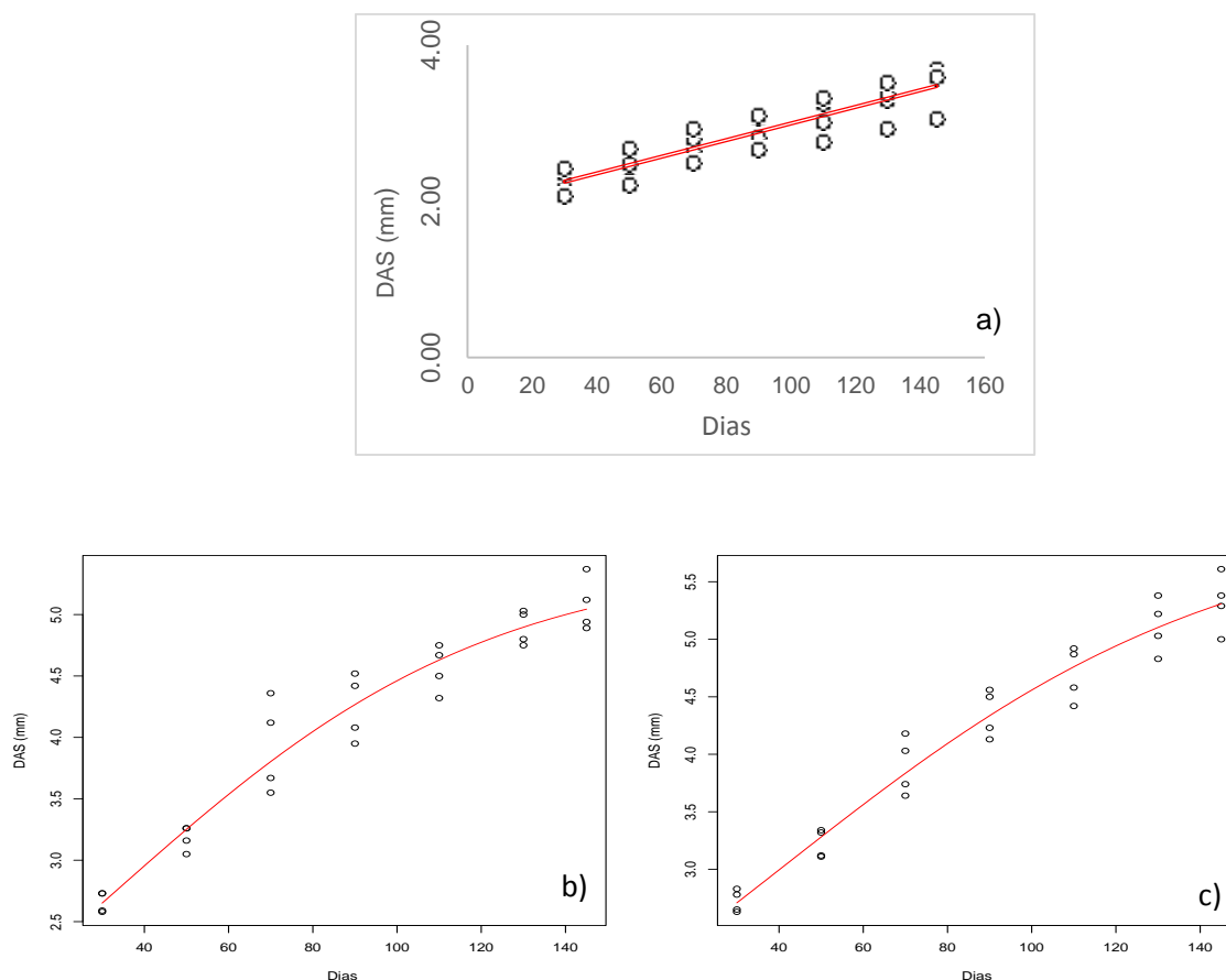
Figura 8. Diâmetro das mudas de Simarouba amara Aubl. em função do tempo de permanência no viveiro. Equações ajustadas para os recipientes de a) 55cm 3 Das = 0,0106x + 1,9322 ( R^2=0,81 ); b) 180 cm 3 Das=5,460063/(1+EXP(0,723901+(X*-0,022206))) ( R^2=0,94 ); c) 280cm 3 Das = 6,044715/(1+EXP(0,777892+(X*-0,018983))) ( R^2=0,96 ). Sendo: Das = diâmetro a altura do colo, x = períodos de permanência no viveiro e R2 = coeficiente de determinação.
