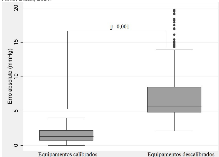
Figura 20. Erro médio absoluto dos esfigmomanômetros calibrados e descalibrados (Boxplot), Santo Antônio de Jesus, Bahia, 2020.
