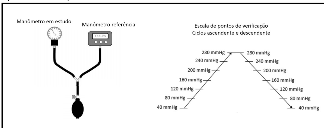
Figura 8. Esquema de montagem do manômetro de referência e escalas de verificação ascendente e descendente – etapa do erro de indicação.
