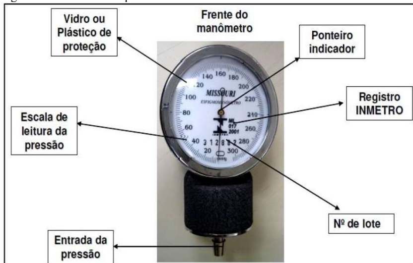
Figura 4. Manômetro de pressão modelo aneróide.
