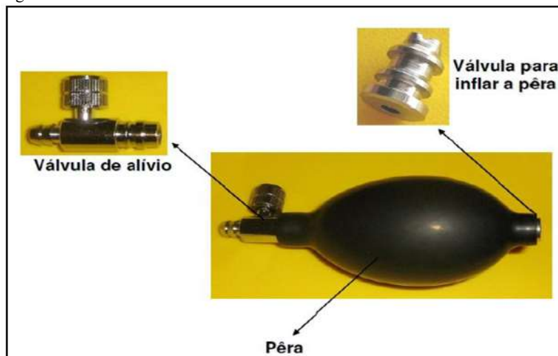
Figura 3. Pera Insufladora.
